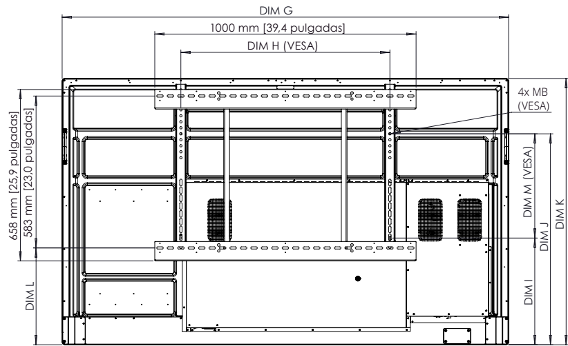
Vista posterior
